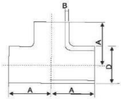
R型三通
