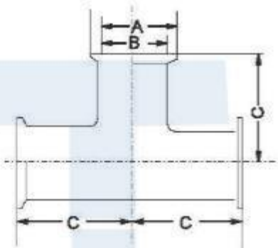
快装三通
