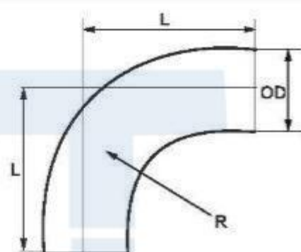
加长弯头
