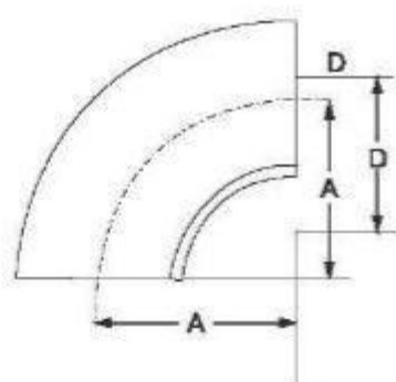
焊接弯头
