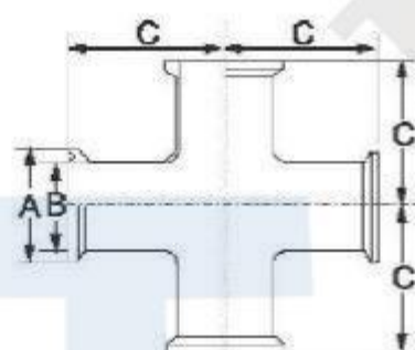
快装四通
