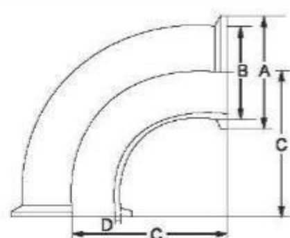
快装弯头
