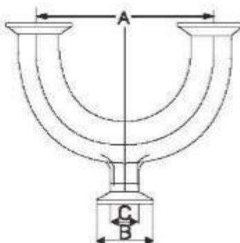
焊接式
